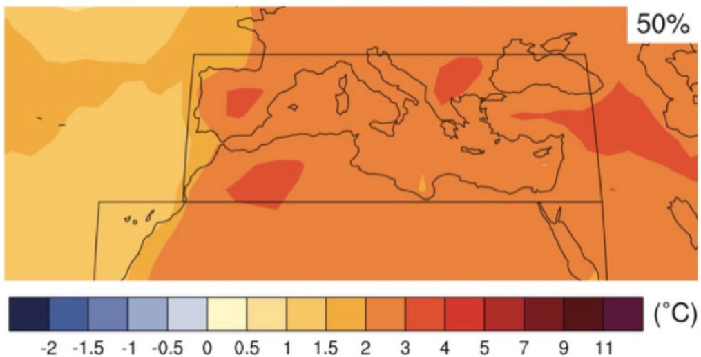
Changement de température en 2081-2100: juin-août, RCP4.5
